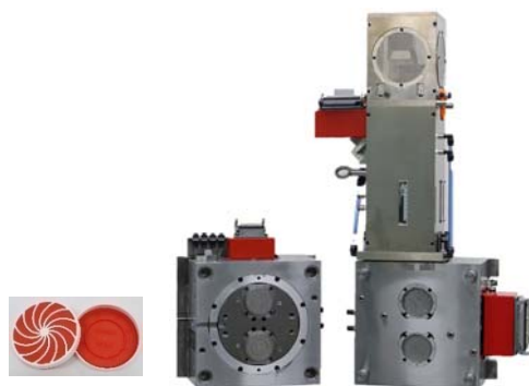
汎用成形機で2色成形を可能にする”BOX INJECTOR”
